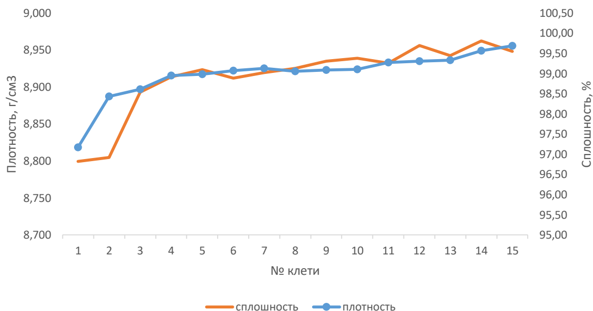
Рис. 2. Зависимость распределения сплошности и плотности по клетям прокатного стана для комплекта №1
