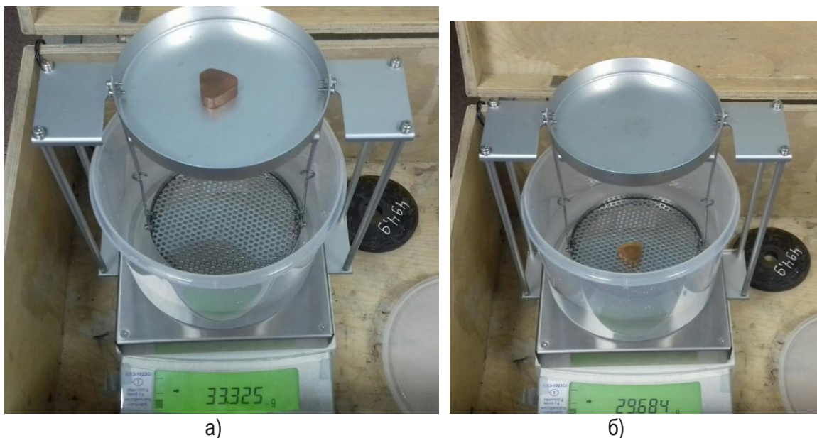
Рис. 1. Измерения массы образцов в воздухе (а) и в жидкости (б)
