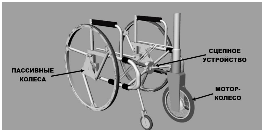
Рис.3. 3D модель ходовой части инвалидной коляски с мотор-колесом тянущего типа и пассивными амортизированными колесами
