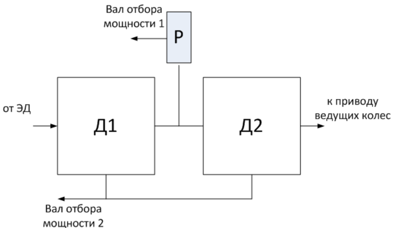
Рис. 3. Комбинированная кинематическая схема работы КП
