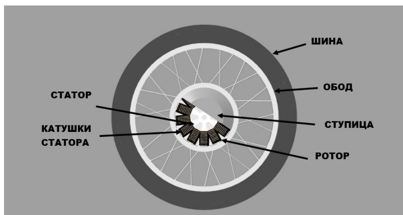
Рис. 1. 3D модель ступичного мотор-колеса Bikight
