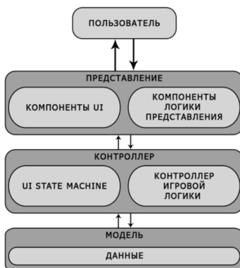
Рис. 1. Схема архитектуры игрового приложения
