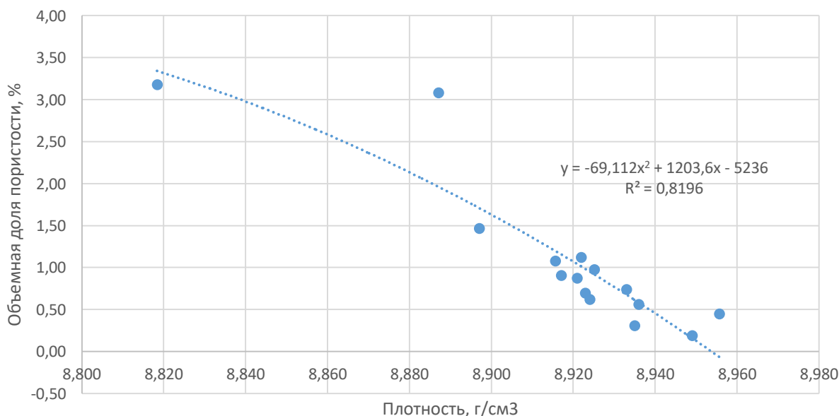
Рис. 4. Взаимосвязь пористости и плотности для комплекта №1
