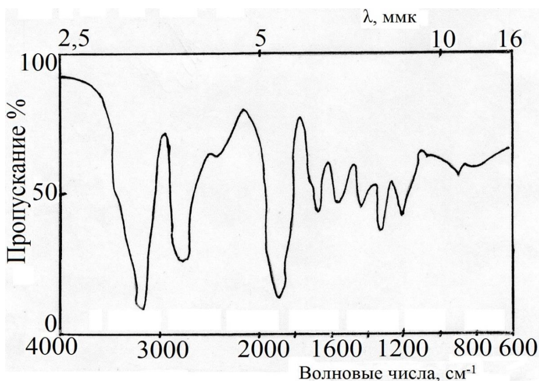
Рис. 2. ИК спектры смесей жирных кислот липидов водоросли Polysiphonia caspica (в жидкой пленке)
