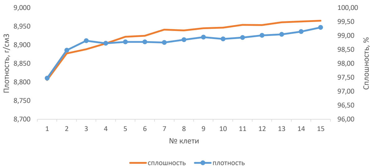
Рис. 3. Зависимость распределения сплошности и плотности по клетям прокатного стана для комплекта №2
