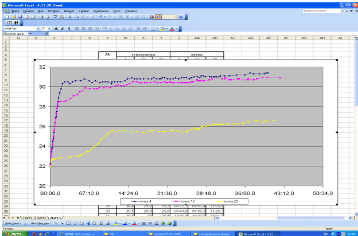
Рис. 6. График диагностических параметров
