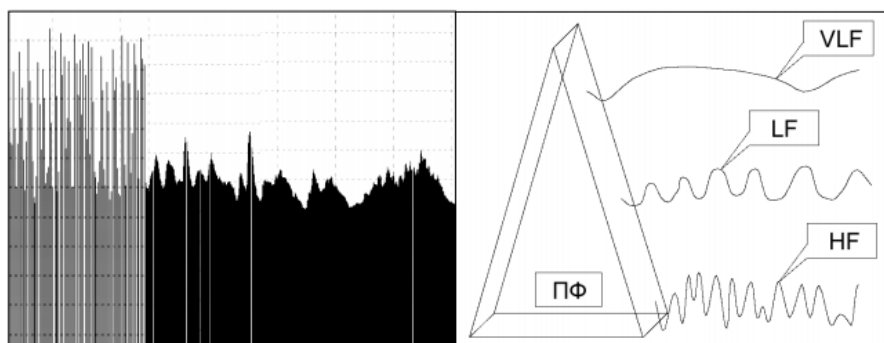
Рис. 5. Спектральный анализ ВСП. Пример кардиоритмограммы
