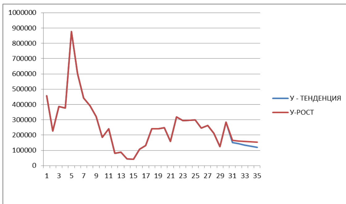
Рис.1. Диаграмма функций Тенденция и Рост
