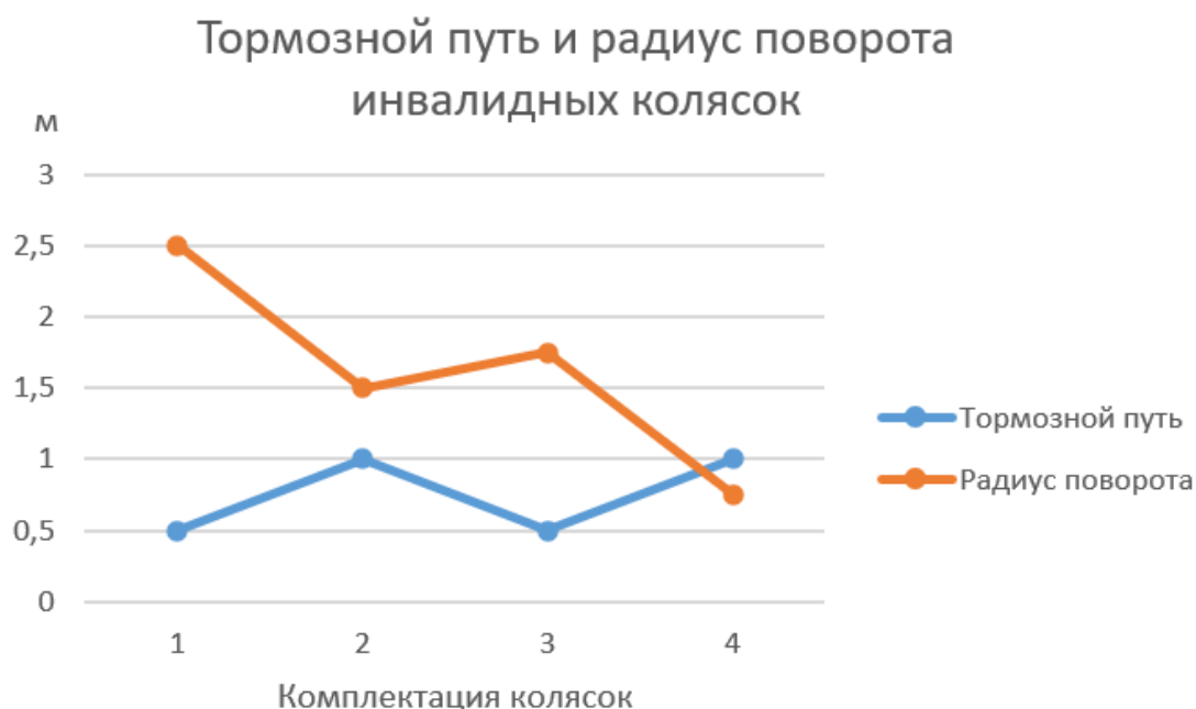
Рис. 5. Радиус поворота и тормозной путь инвалидных колясок различных комплектаций
