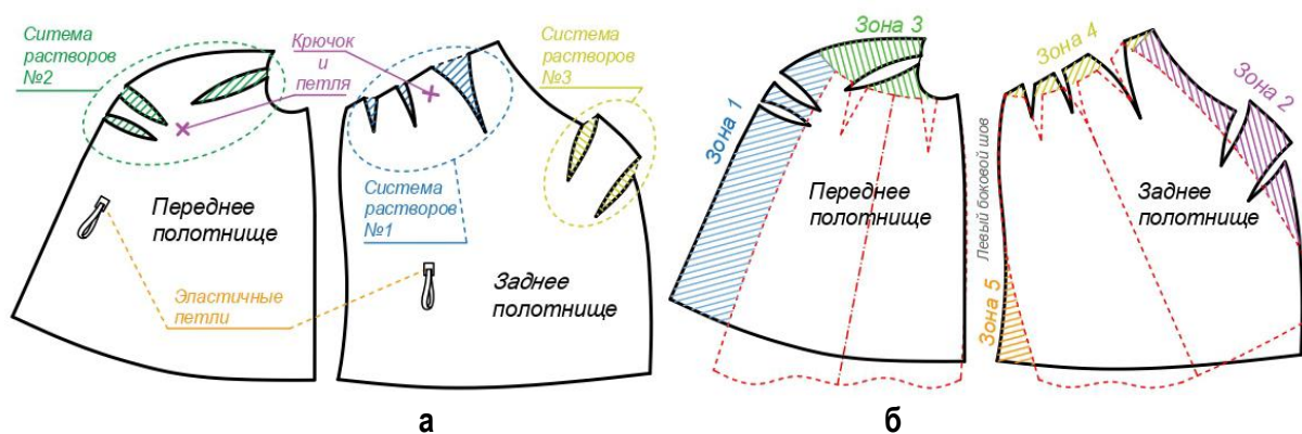
Рис. 3. Чертежи конструкции юбок для верховой езды XIX в. с отмеченными конструктивными особенностями: а – системы вытачек; б – избыточная ширина деталей
