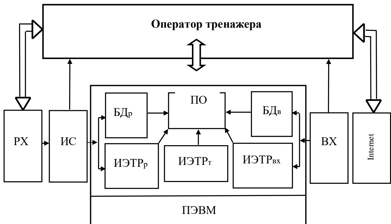
Рис. 1. Функциональная схема виртуального тренажера
