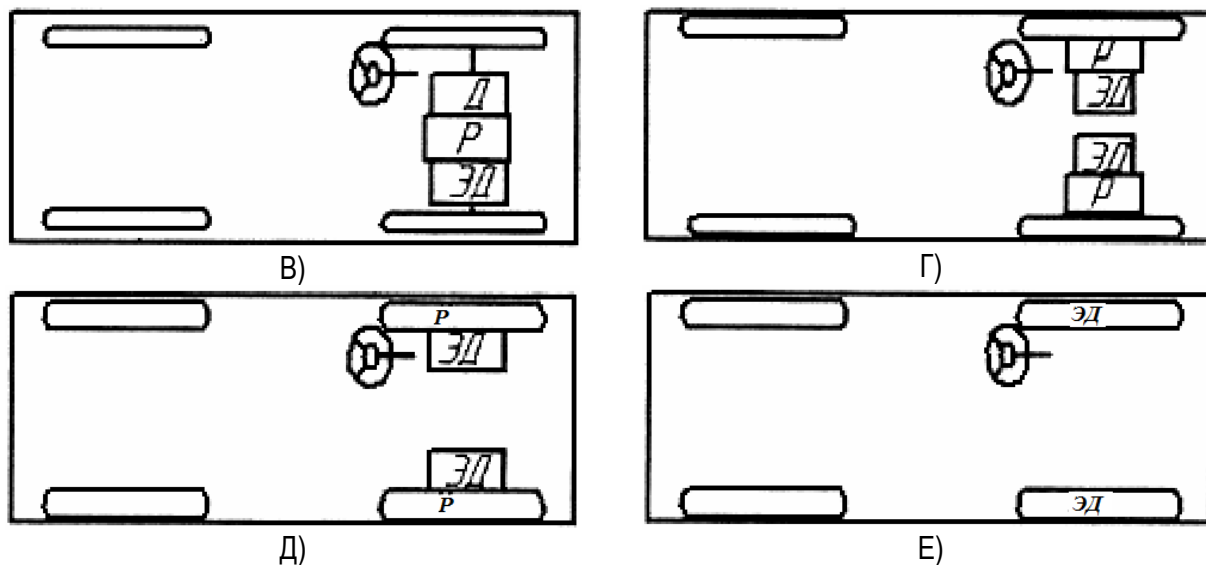
Рис. 1. Варианты компоновочных схем ТЭПА
