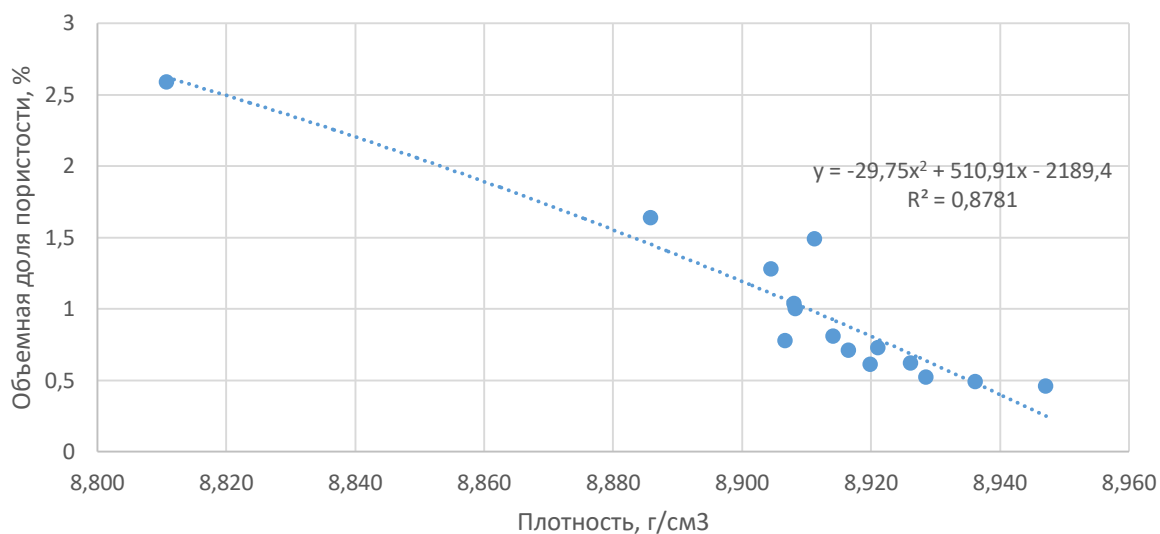
Рис. 5. Взаимосвязь пористости и плотности для комплекта №2
