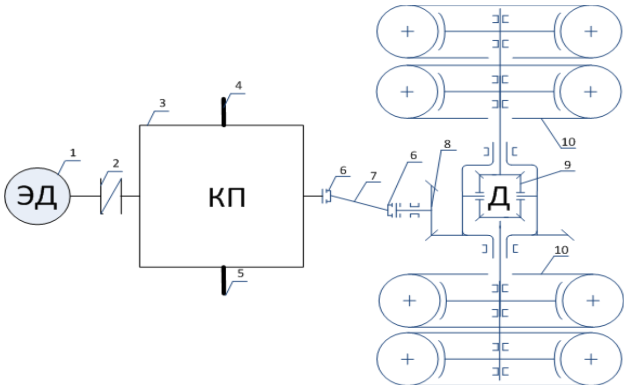
Рис. 2. Кинематическая комбинированная схема ТЭПА
