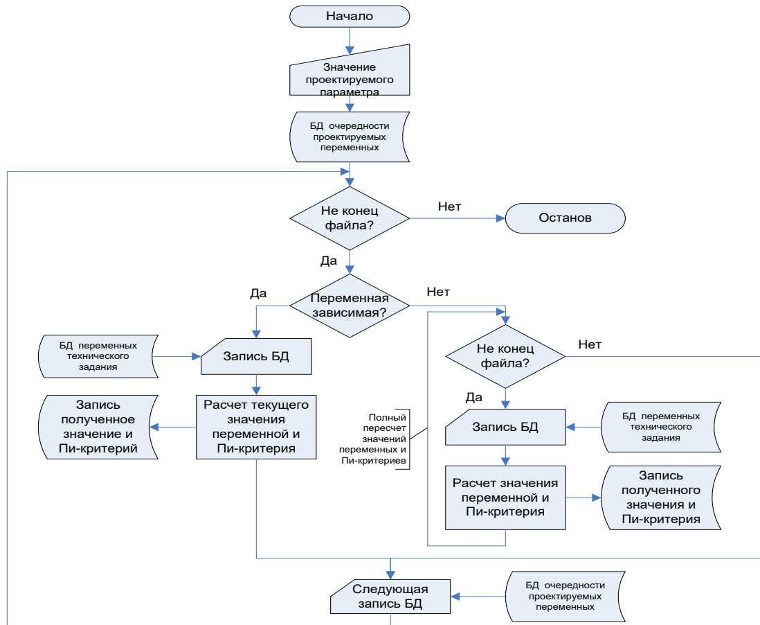
Рис. 5. Блок-схема расчета проектируемых значений переменных
