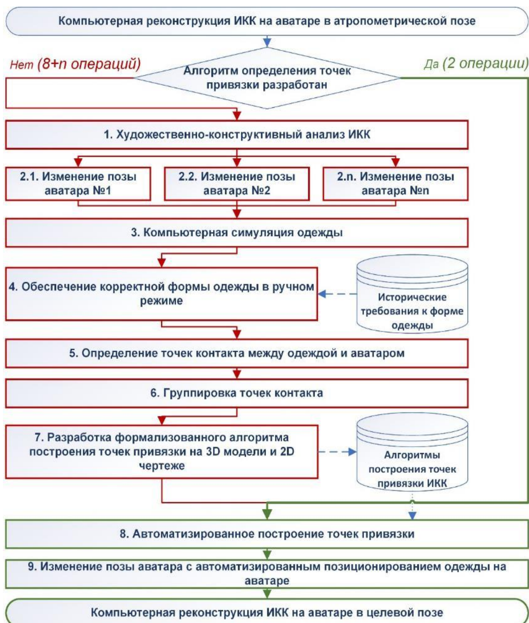
Рис. 1. Блок-схема процесса преобразования статичного виртуально костюма в динамичный
