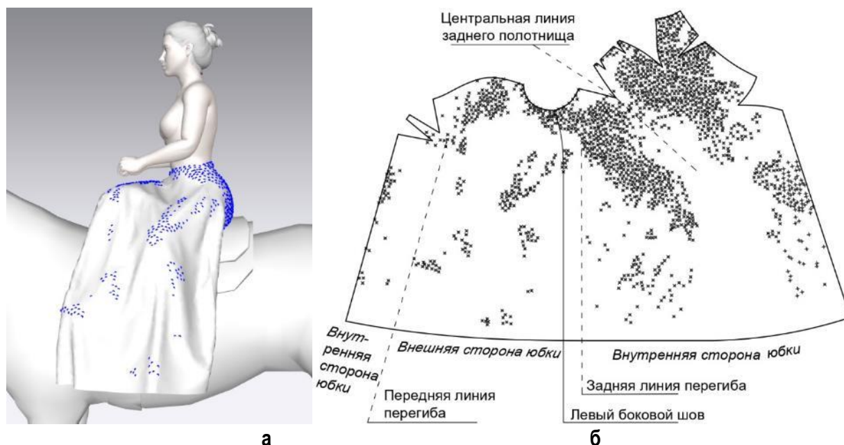
Рис. 5. Определение точек контакта между юбкой ИКК и аватаром всадницы: а – 3D модель; б – 2D чертеж
