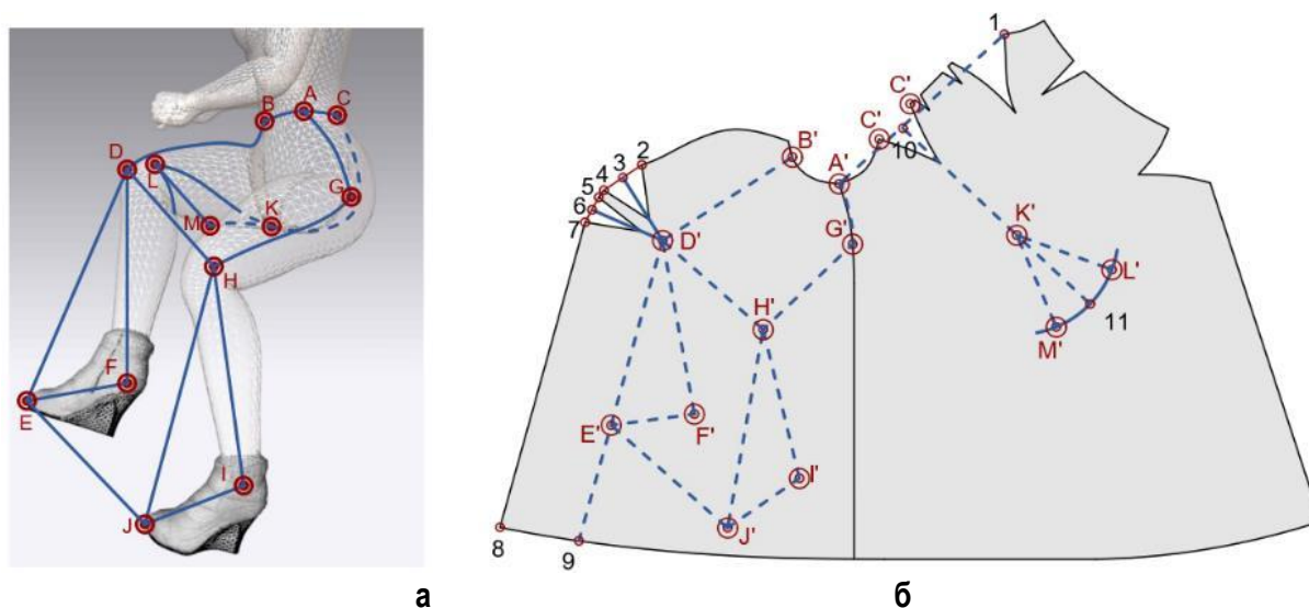
Рис. 7. Точки привязки юбки ИКК для верховой езды к аватару: а – на 3D модели ( A...M ); б – на чертеже конструкции ( A'...M' )
