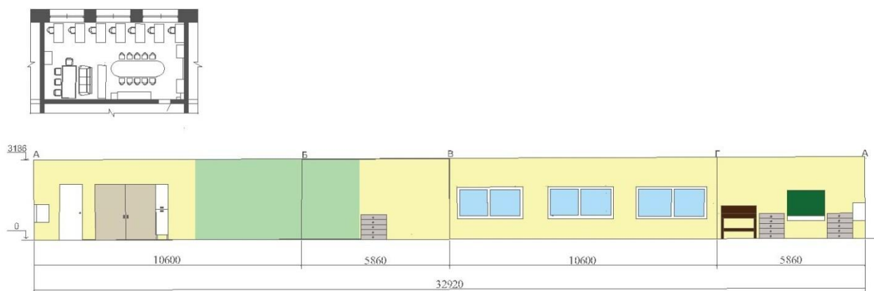
Рисунок Б.4 – Развертка стен аудитории №1211
