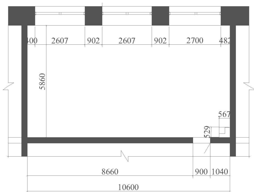
Рисунок А.6 – Обмерный план аудитории №1211, М 1:100
