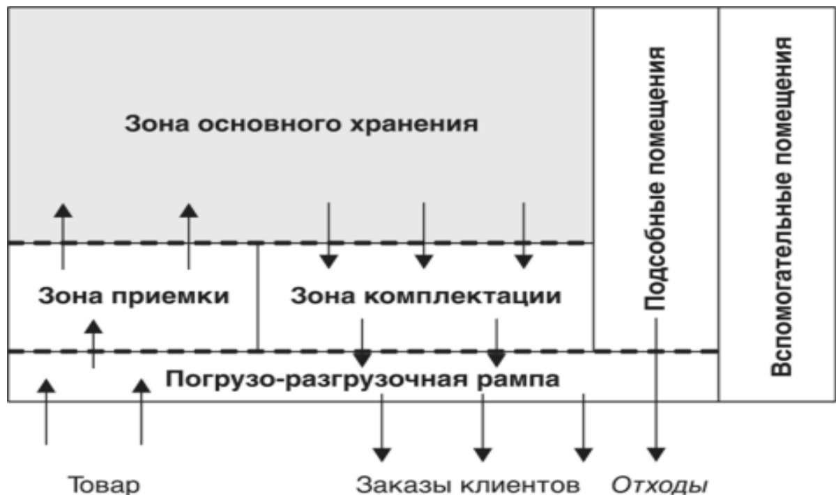
Рисунок 3 - План склада компании «Абсолют»
