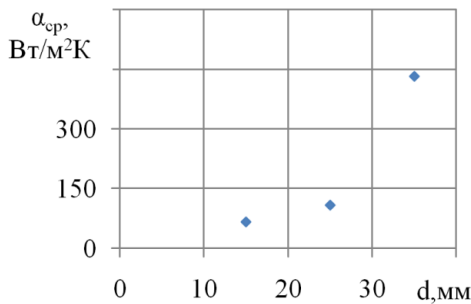
Рисунок 10 – Распределение среднего коэффициента теплоотдачи в зависимости от диаметра трубы
