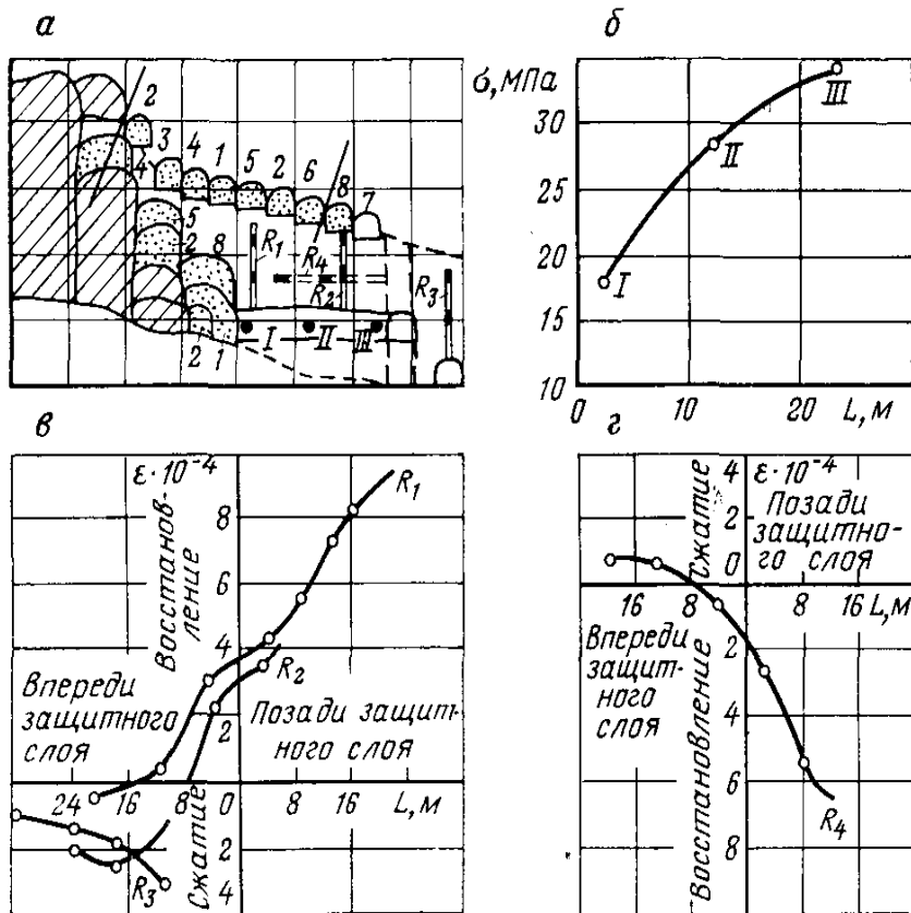
Рис. 1. Исследование напряженно-деформированного состояния массива: а — динамика развития горных работ (цифры 1—8 показывают порядок отработки камер), схема расположения измерительных скважин (I, II, III) и станций глубинных реперов ( R_1 — R_4 ); б — результаты измерения напряжений в скважинах I, II, III; в, г — результаты измерения деформаций соответственно в вертикальном и горизонтальном направлениях; L — расстояние до очистной выемки; а — относительные деформации
