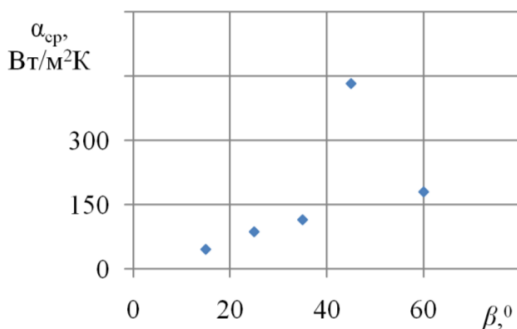
Рисунок 8 – Распределение среднего коэффициента теплоотдачи в зависимости от угла наклона лопаток
