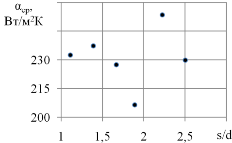
Рисунок 5 – Распределение среднего коэффициента теплоотдачи от безразмерного шага.
