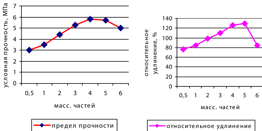
Рис. 1. Зависимость физико-механических свойств композиции от количества сшивающего агента БЦС
