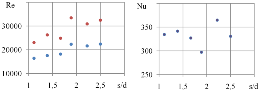
Рисунок 6 – Влияние безразмерного шага на: а) число Рейнольдса на входе и выходе из трубы, б) число Нуссельта.
