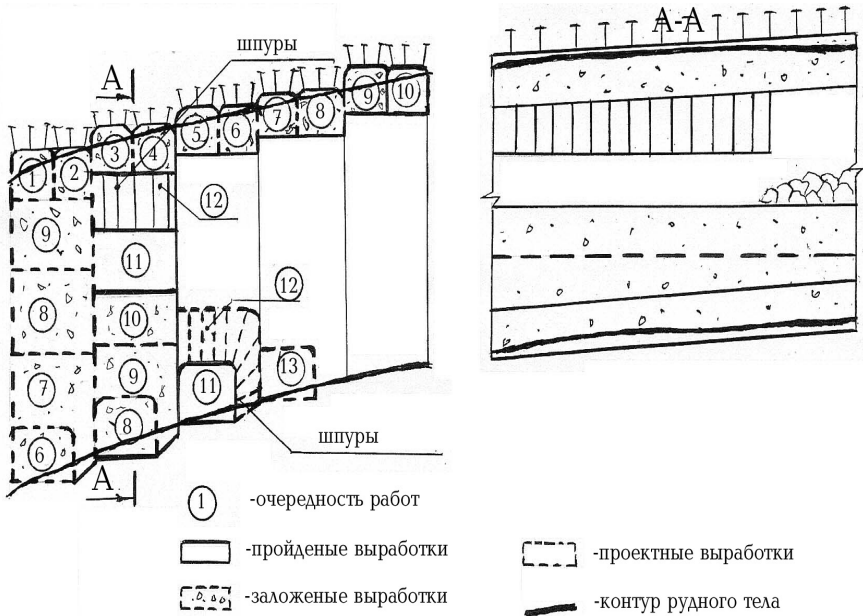
Рис. 2. Вариант слоевой системы разработки
