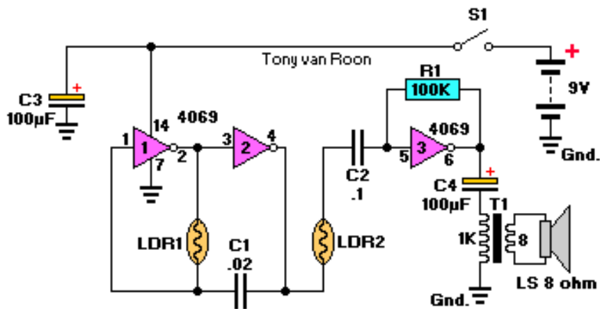
Рис.1. Принципиальная электрическая схема терменвокса
