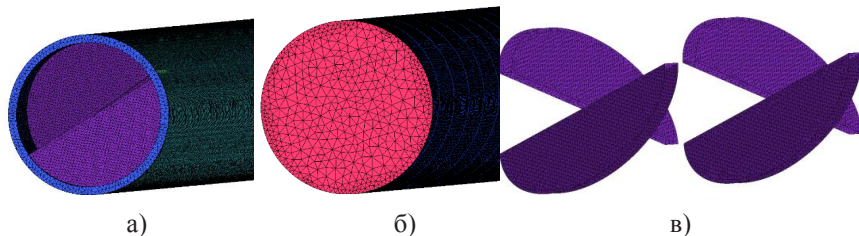
Рисунок 3 – Сеточная модель: а) твердого тела, б) проточной части, в) скрещенные ребра.
