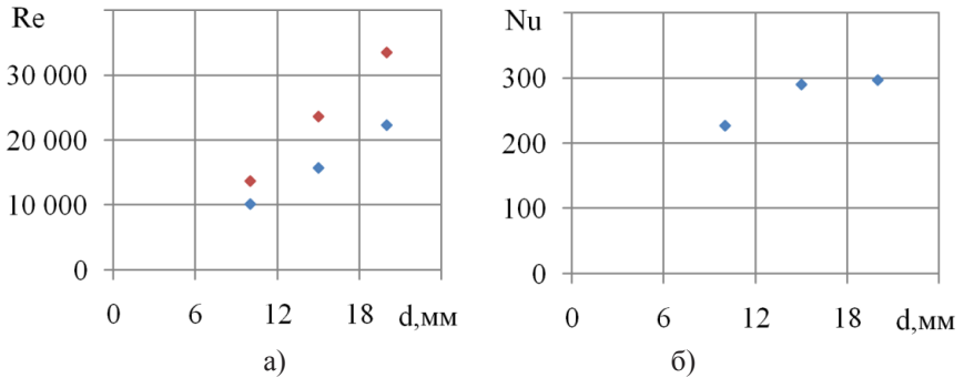
Рисунок 9 – Влияние безразмерного шага на: а) число Рейнольдса на входе и выходе из трубы, б) число Нуссельта.
