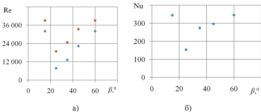
Рисунок 7 – Влияние безразмерного шага на: а) число Рейнольдса на входе и выходе из трубы, б) число Нуссельта.
