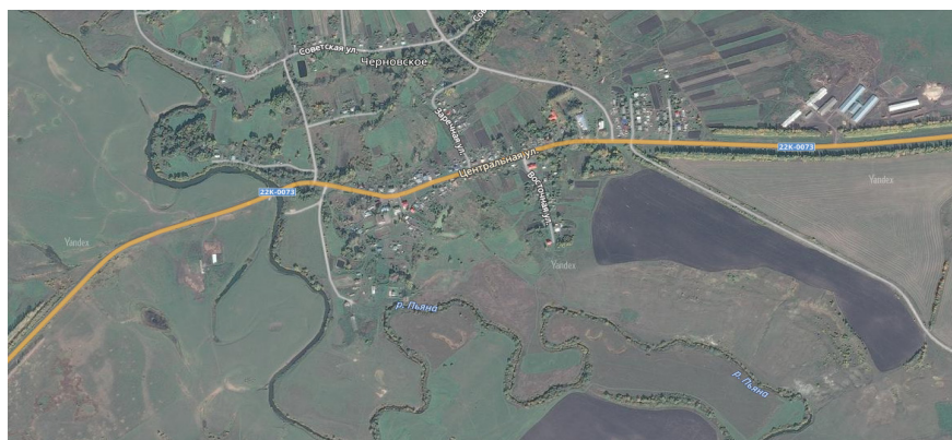
Рис. 1. Местоположение геологического обнажения
