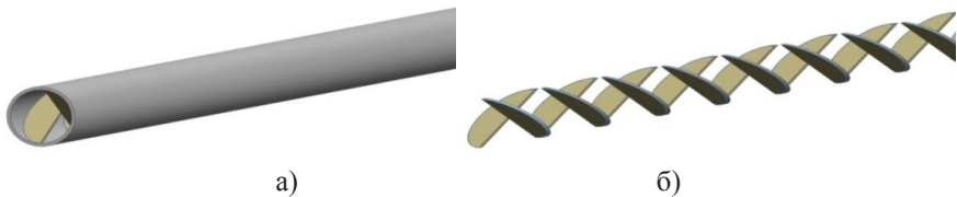
Рисунок 1 – Модель цилиндрического канала: а) общий вид трубочки, б) скрещенные ребра.
