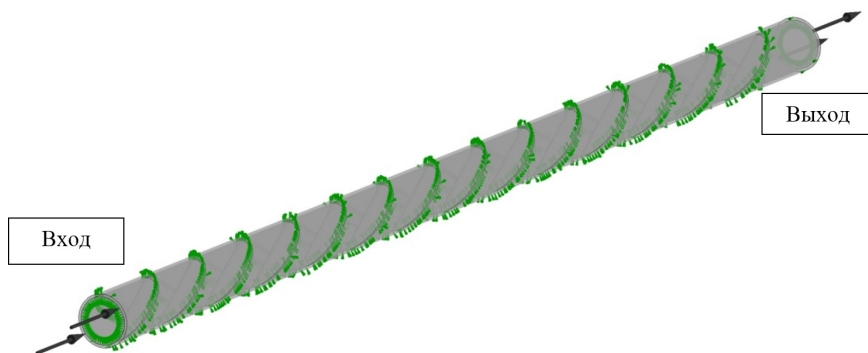
Рисунок 4 – Схема приложения граничных условий.
